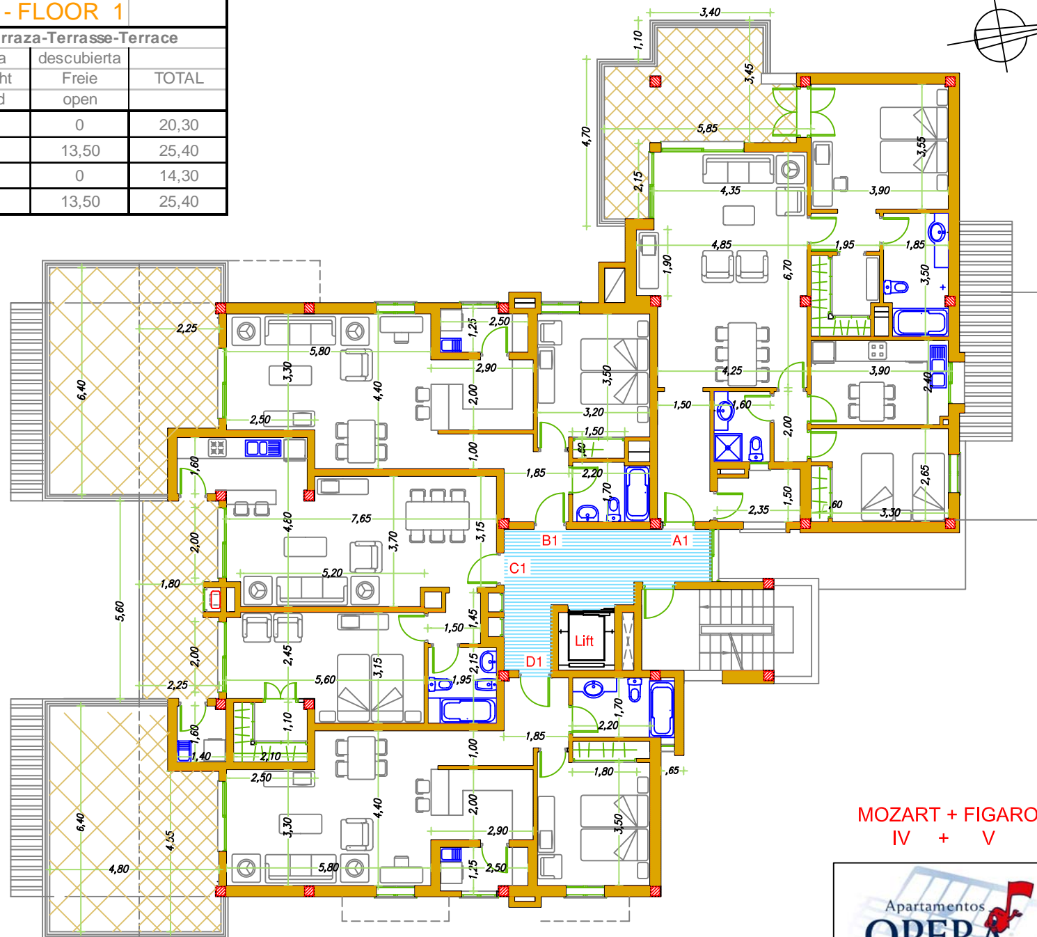
PLANTA - STOCKWERK - FLOOR 1
