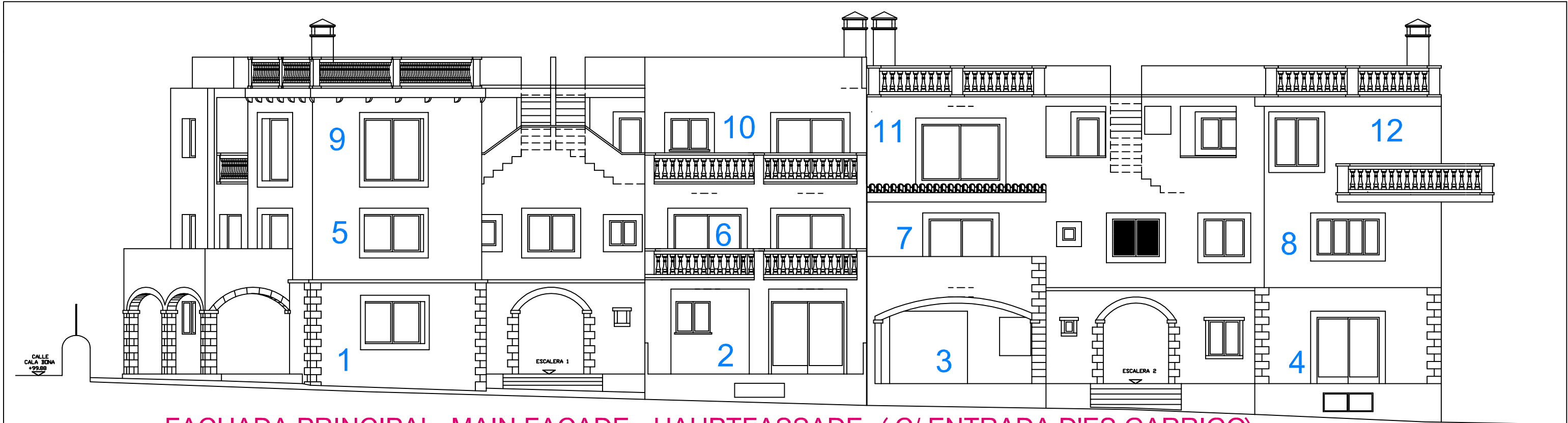
FACHADA PRINCIPAL- MAIN FACADE - HAUPTFASSADE ( C/ ENTRADA D'ES GARRIGO) << ELS ROSSINYOLS >>
